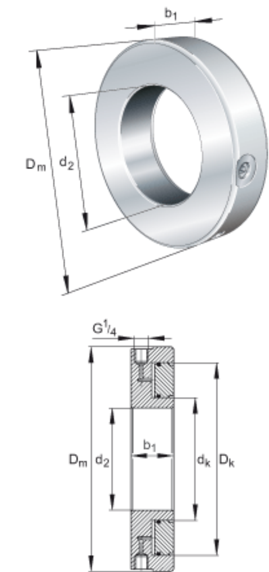
FAG HYDNUT100-HEAVY图片
